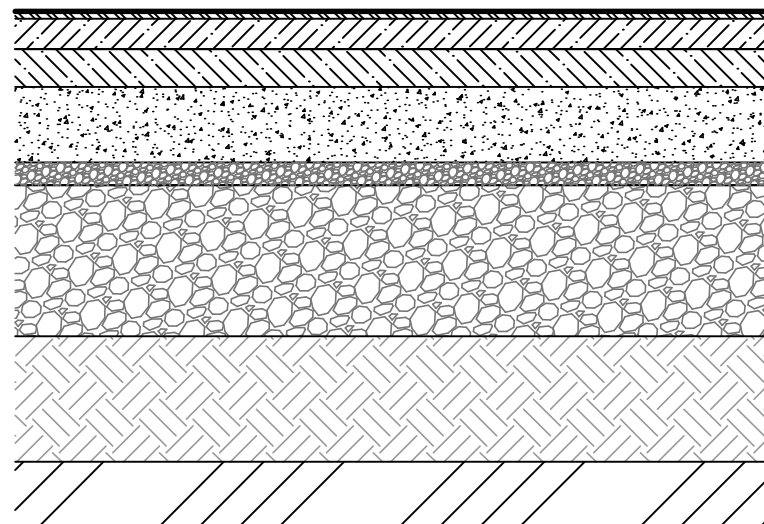
Skladba hřiště
