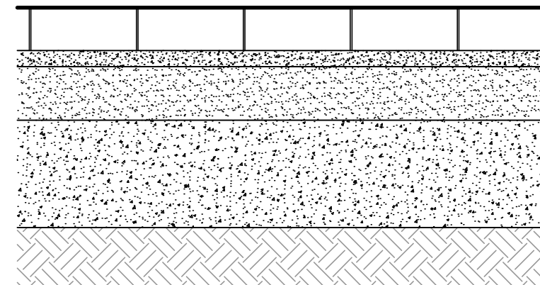
Skladba chodníku – s pojezdem
